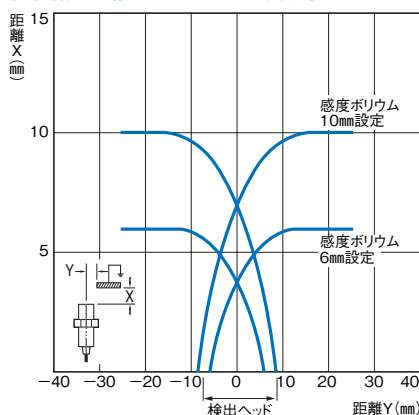
検出領域(接地された金属板)
