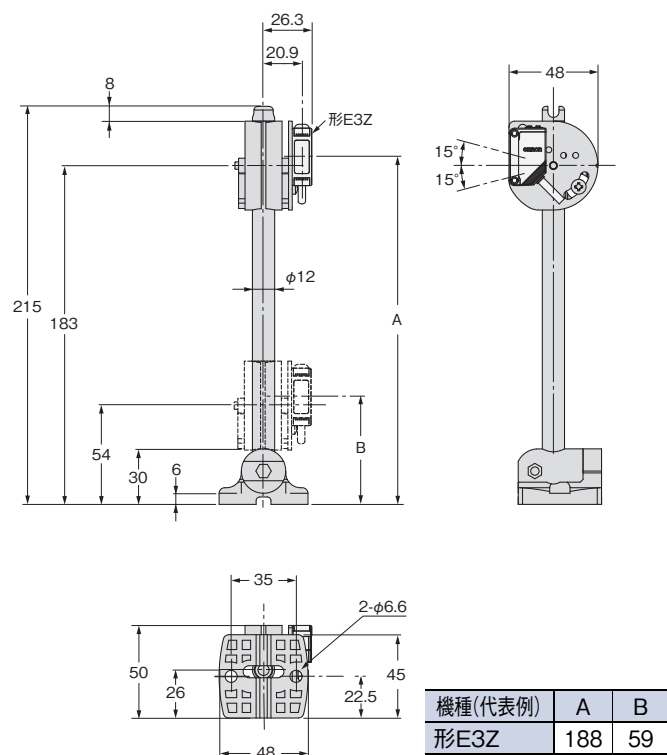
形E39-L93FH
