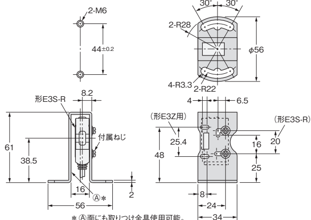
形E39-L98
