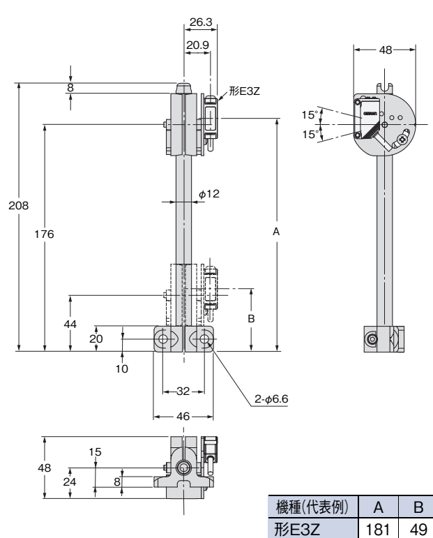
形E39-L93V
