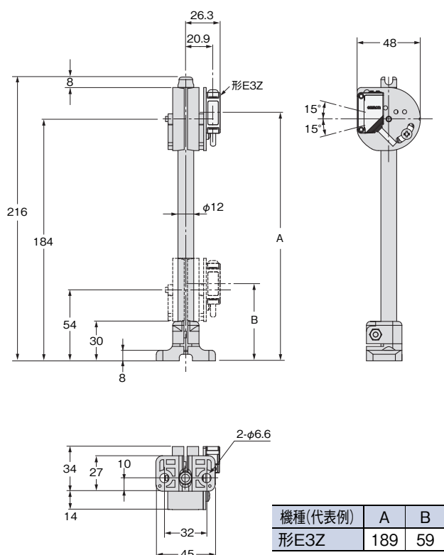
形E39-L93H
