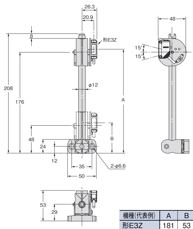
形E39-L93FV
