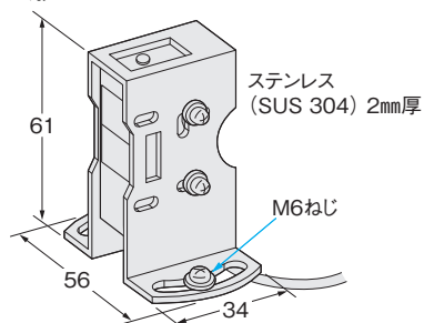
形E39-L98
