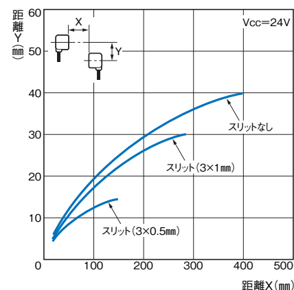
平均移動特性 形EE-SPW321/421
