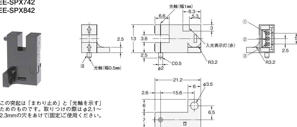
端子配置
