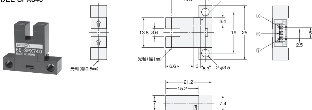
端子配置
