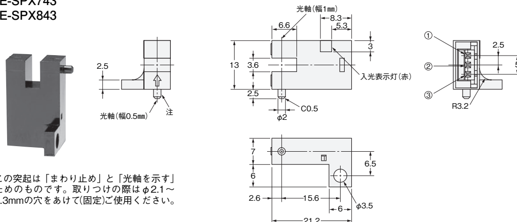
端子配置
