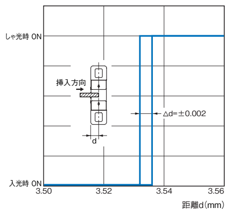
繰り返し検出位置特性 形EE-SX970
