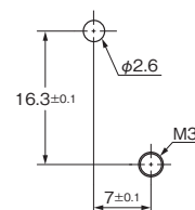
取りつけ穴加工寸法
