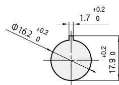
取付パネル有効板厚
