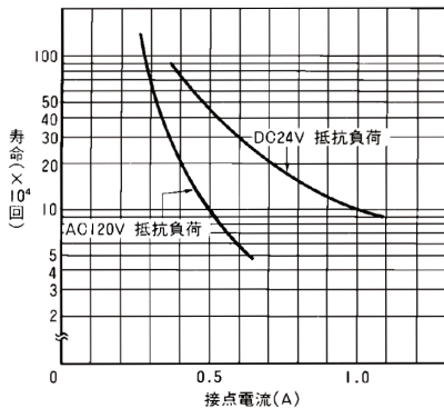
寿命曲線
