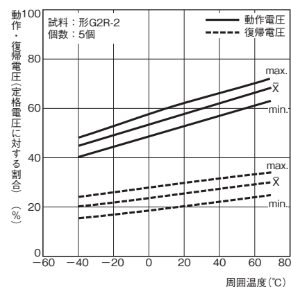
形G2R-2
