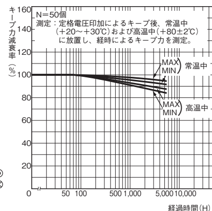
形G2RK-1
