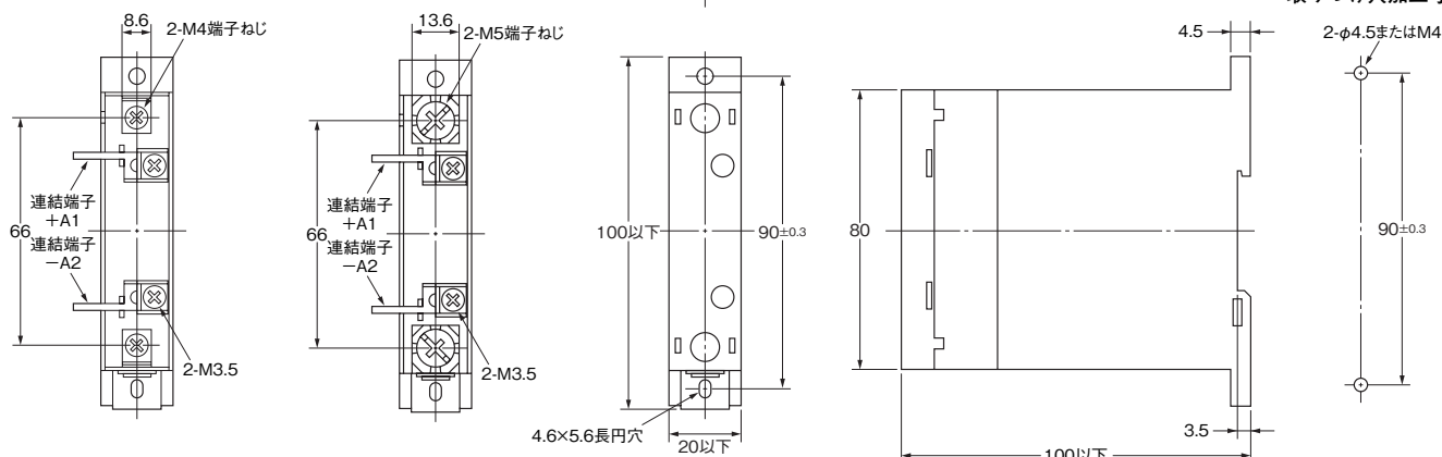
取り付け穴加工寸法
