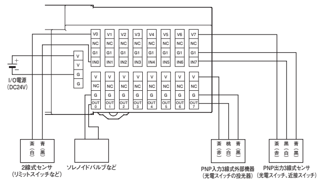
形GX-MD3228(PNP対応)
