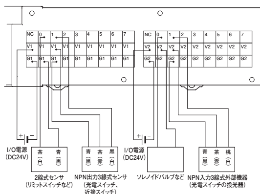
形GX-MD1612(NPN対応)
