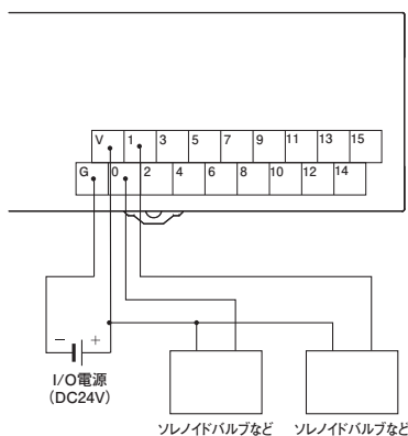
形XWT-OD16(NPN対応)
