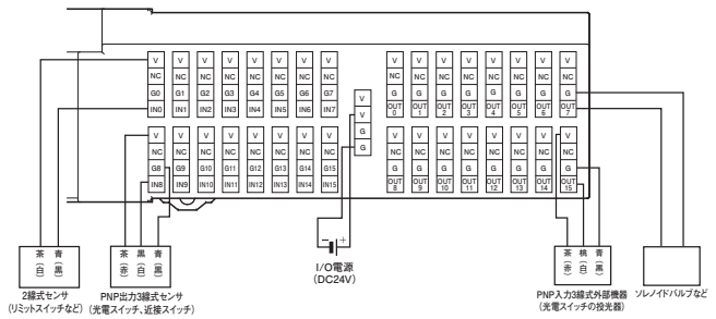
形GX-MD3228(PNP対応)
