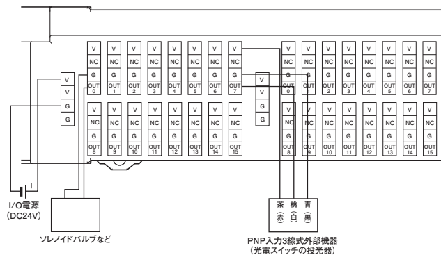
形GX-OD3228(PNP対応)
