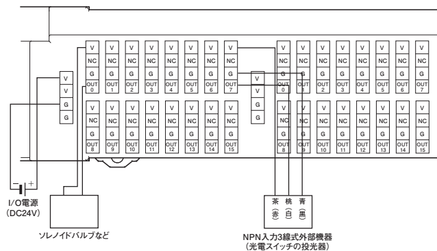
形GX-OD3218(NPN対応)
