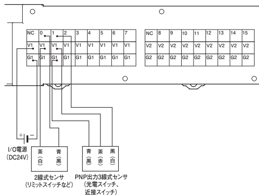
形GX-OD1622(PNP対応)
