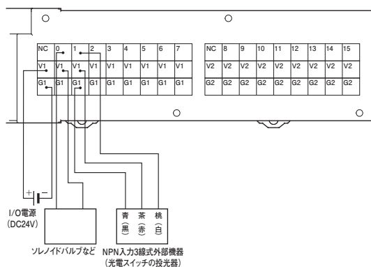
形GX-MD1612(NPN対応)
