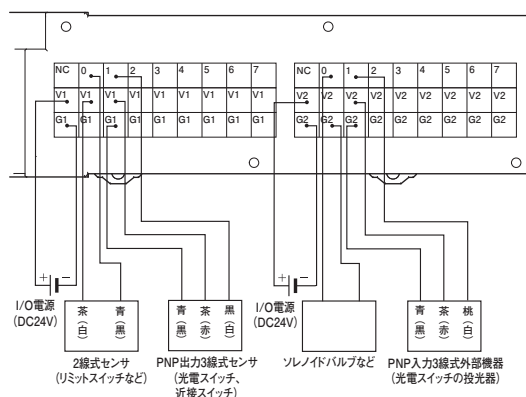
形GX-MD1622(PNP対応)
