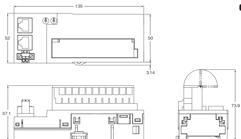
形GX-MD1611/MD1621
