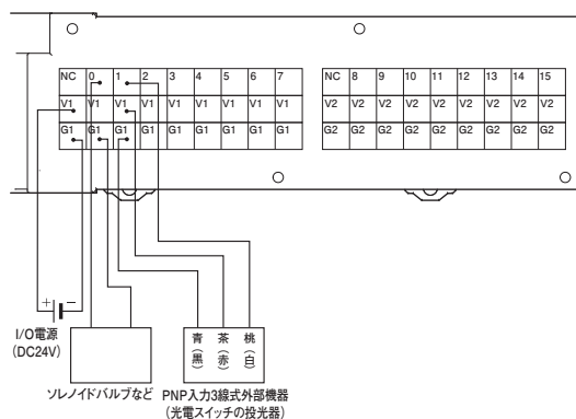
形GX-MD1622(PNP対応)
