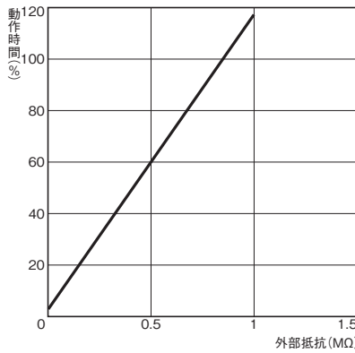
●形H3FA-A/-SA/-AU/-SAU
