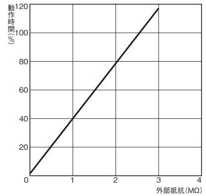
●形H3FA-B/-SB/-BU/-SBU
