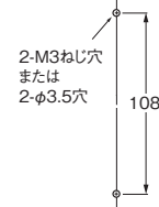
取り付け穴加工寸法
