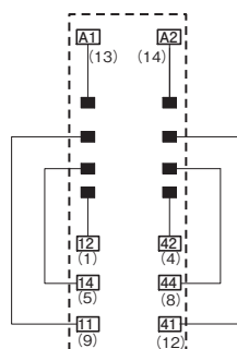
端子配置/内部接続図 (TOP VIEW)
