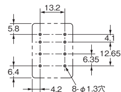
取り付け穴加工寸法
