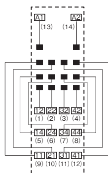
端子配置/内部接続図 (TOP VIEW)
