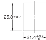
取り付け穴加工寸法
