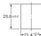
取り付け穴加工寸法
