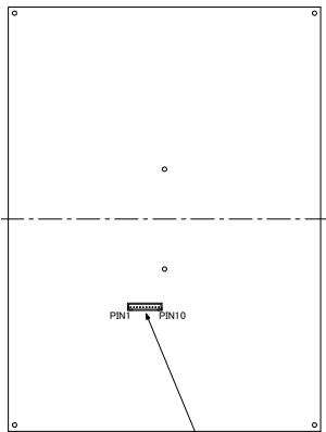
ハウジング XHP-10（JST）
