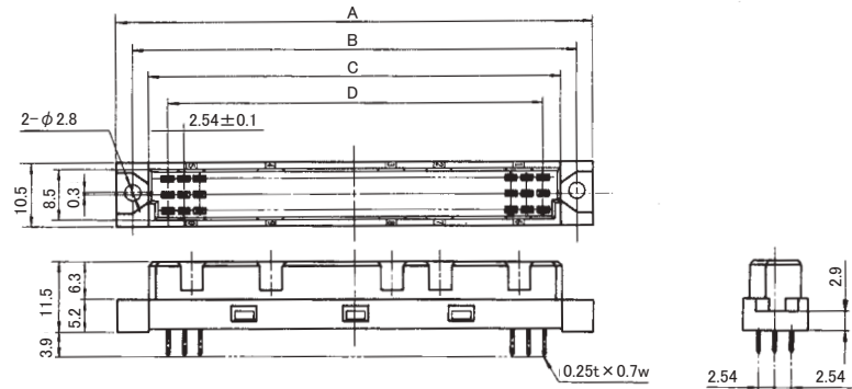
バックボード寸法図
