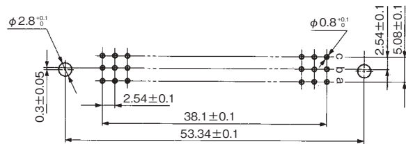
バックボード寸法図
