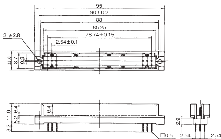
バックボード寸法図
