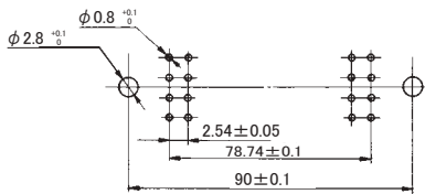
バックボード寸法図
