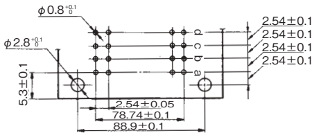
バックボード寸法図
