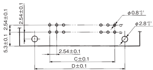
バックボード寸法図
