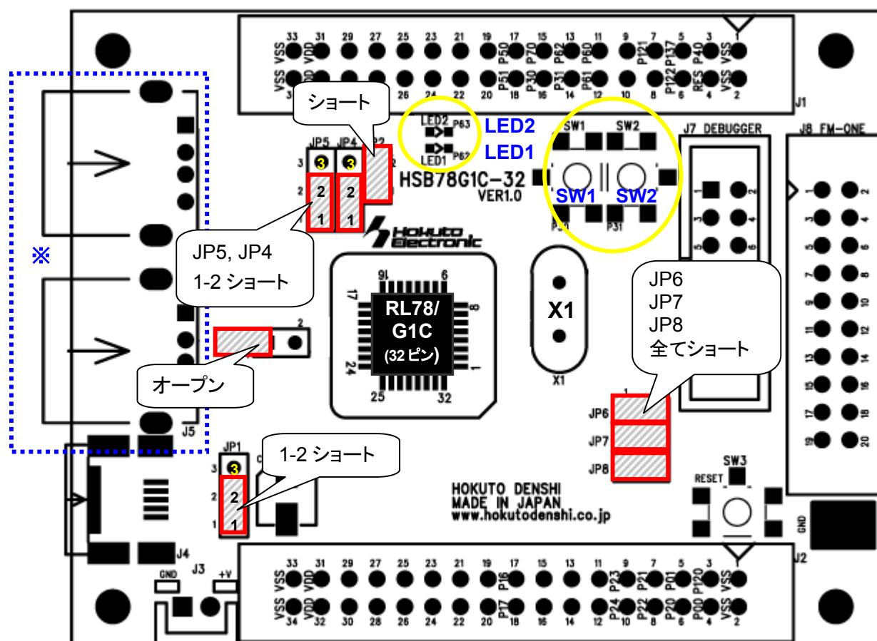
図 4-1 初期設定図
