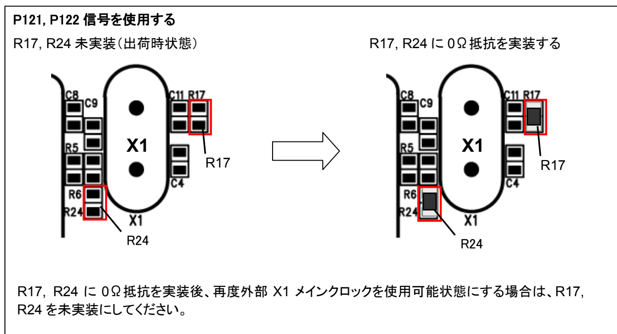
図 2-5 R17, R24 抵抗設定図
