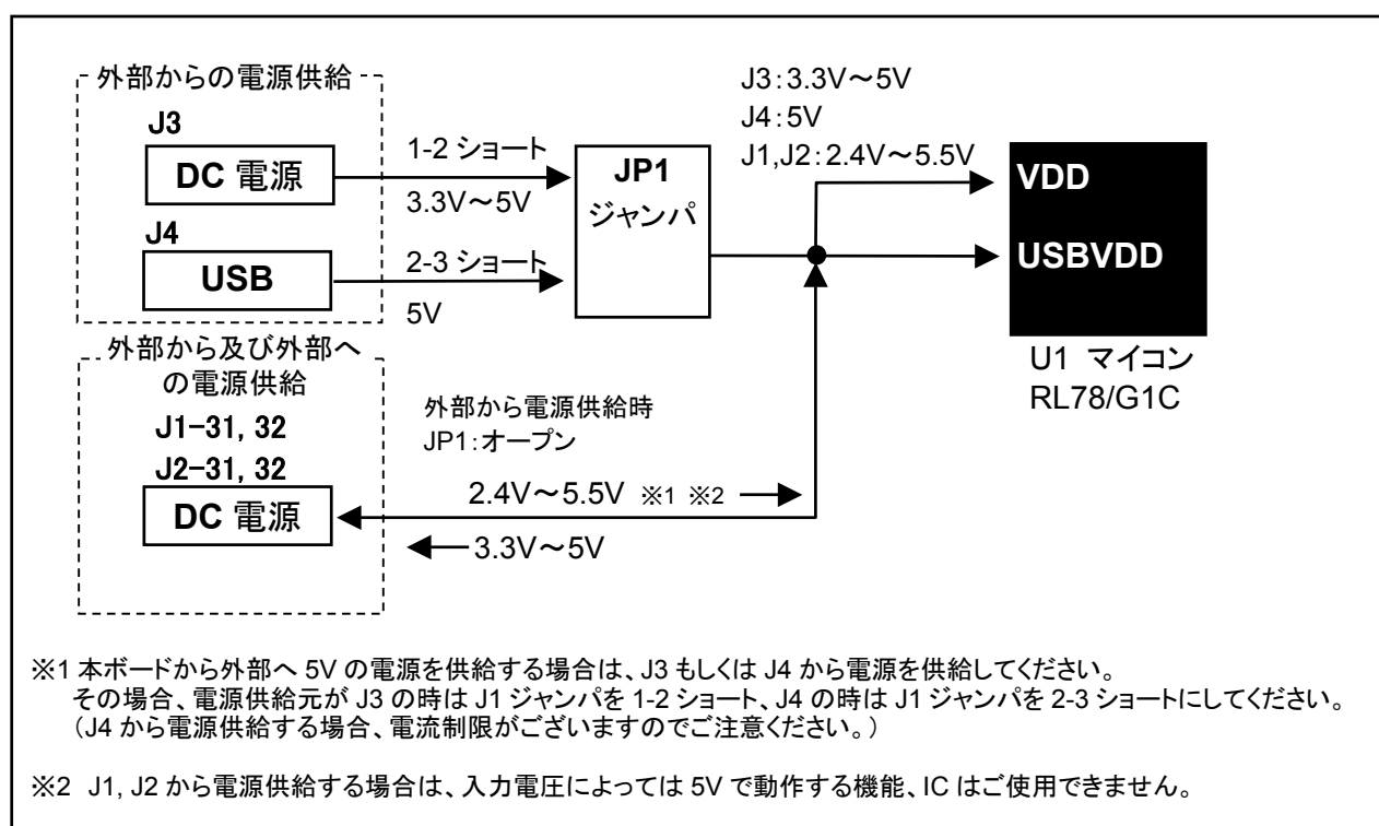
図 2-1 電源供給イメージ図
