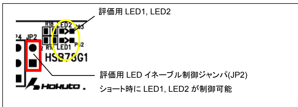
図 2-6 評価用 LED イネーブル制御ジャンパ設定図(JP2)
