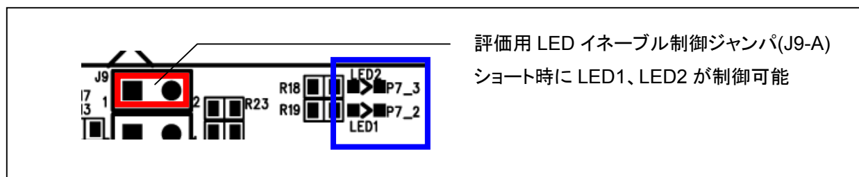
図 4-7 評価用 LED イネーブル制御ジャンパ設定図 (J9-A)
