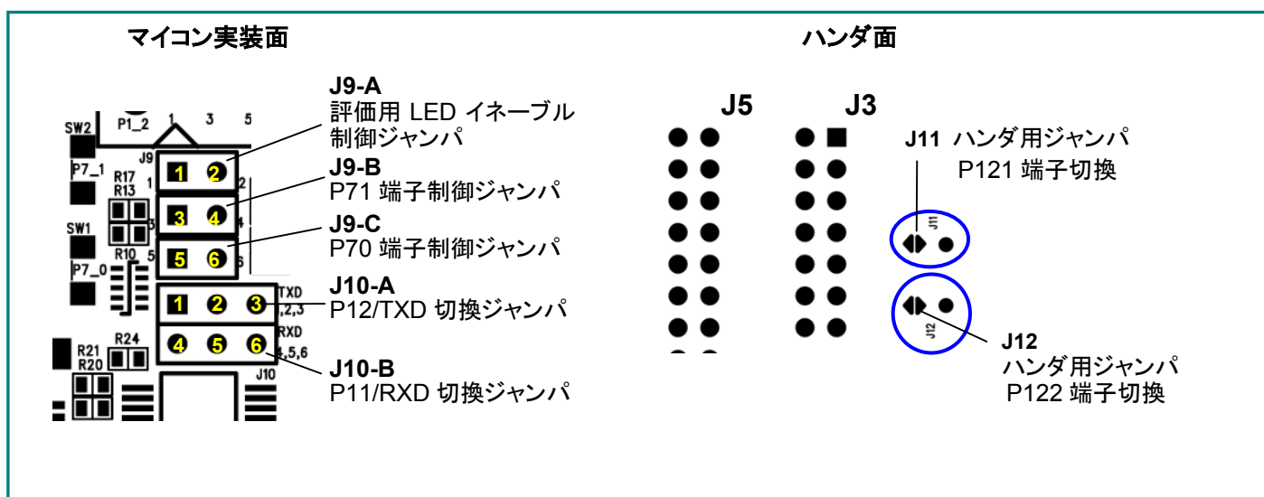
図 3-2 ボード配置補足図
