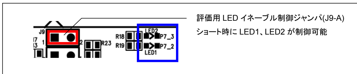
図 4-8 評価用 LED イネーブル制御ジャンパ設定図 (J9-A)
