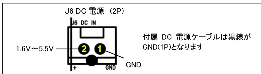
図 4-2 DC 電源図
