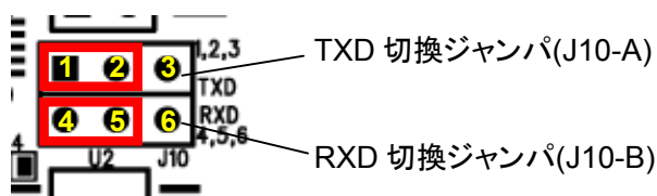
図 2-3 J10-A, J10-B ジャンパ設定例
