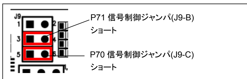
図 2-8 P71, P70 信号制御ジャンパ設定図 (J9-B, J9-C)
