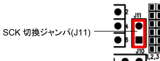
図 2-4 J10-A, J10-B, J11 ジャンパ設定例
