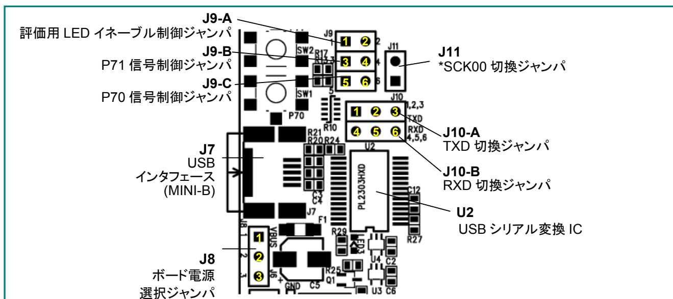
図 1-2 ボード配置補足図
