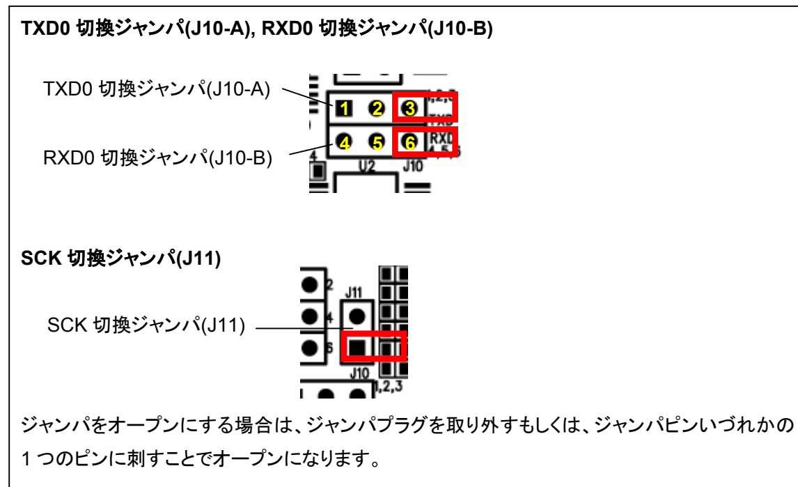
図 2-5 J10-A, J10-B, J11 ジャンパ設定図
