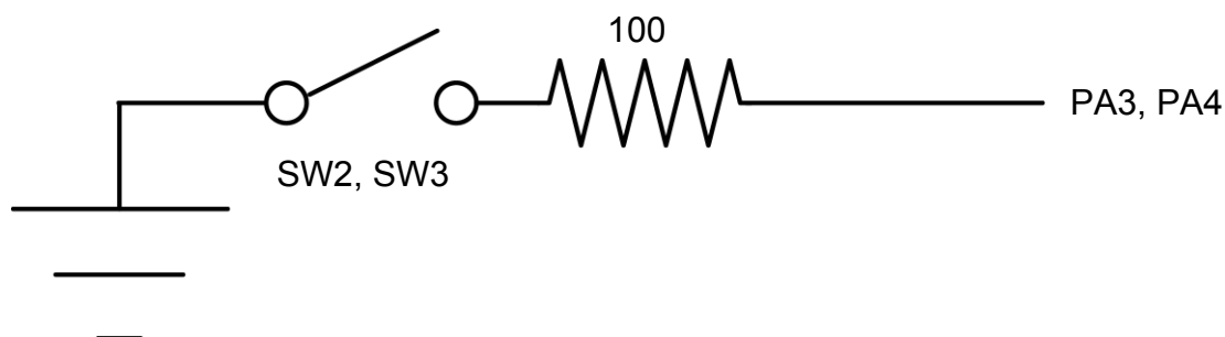
図 4-3 評価用スイッチ回路図
