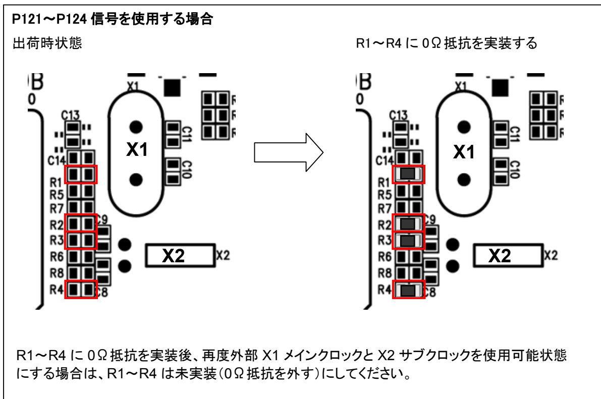
図 2-6 R1～R4 抵抗設定図
