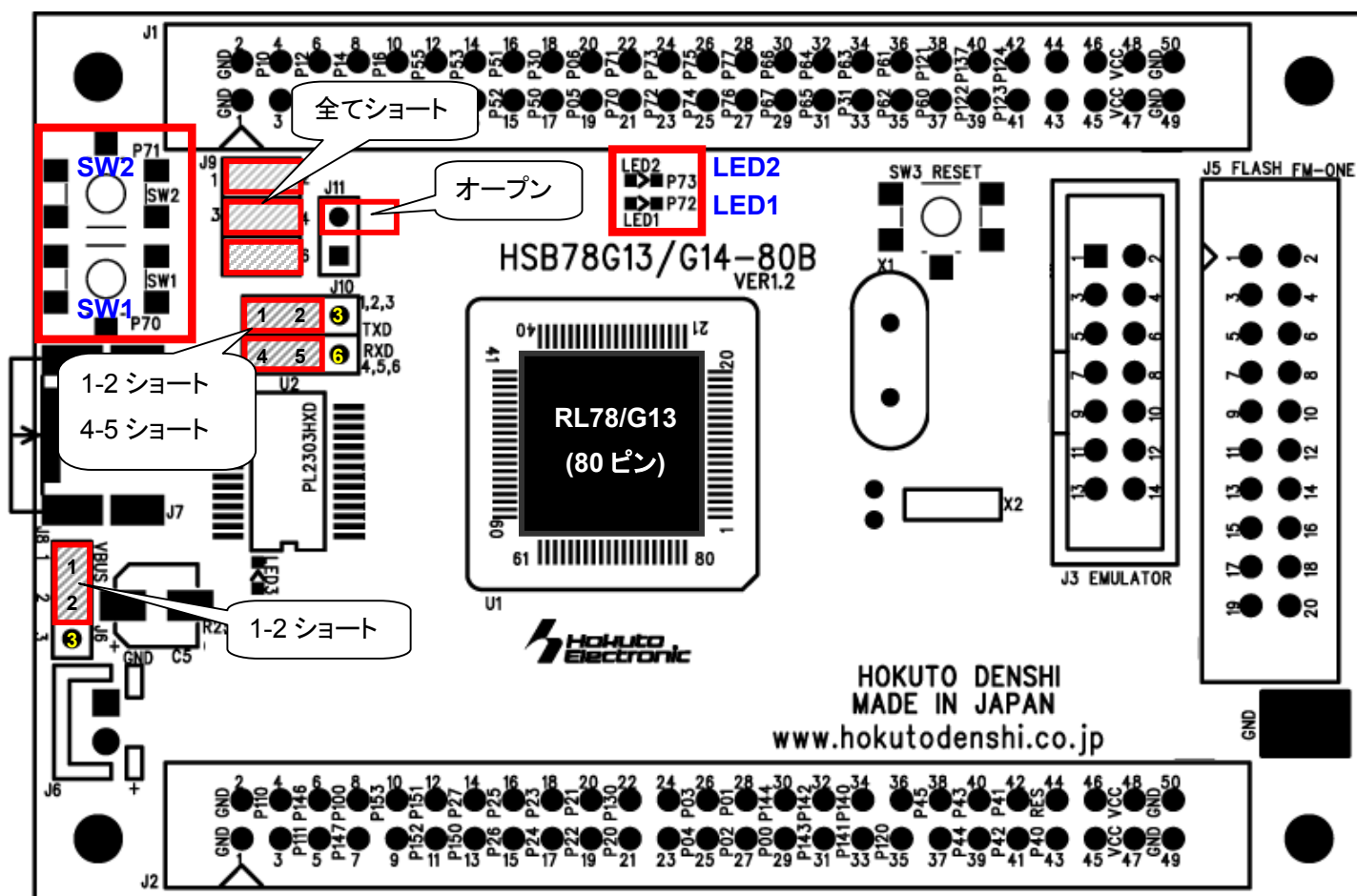
図 4-4 ジャンパピン初期状態図
