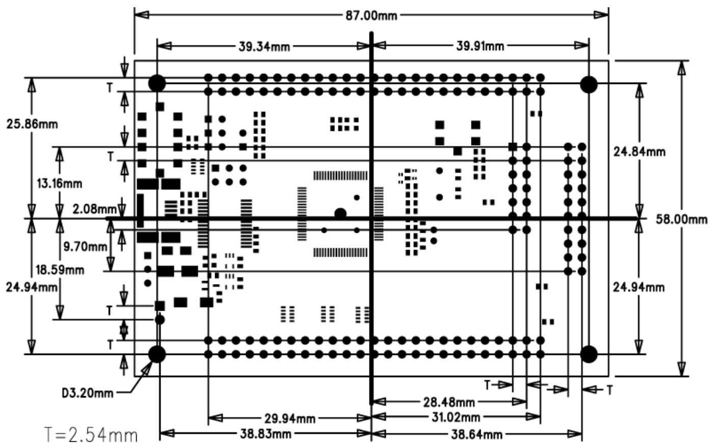
図 4-1 ボード外寸図
