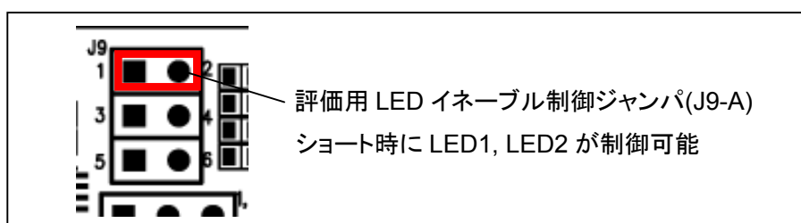
図 2-7 評価用 LED イネーブル制御ジャンパ設定図 (J9-A)
