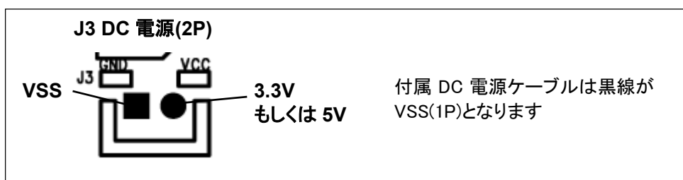
図 2-3 DC 電源図
