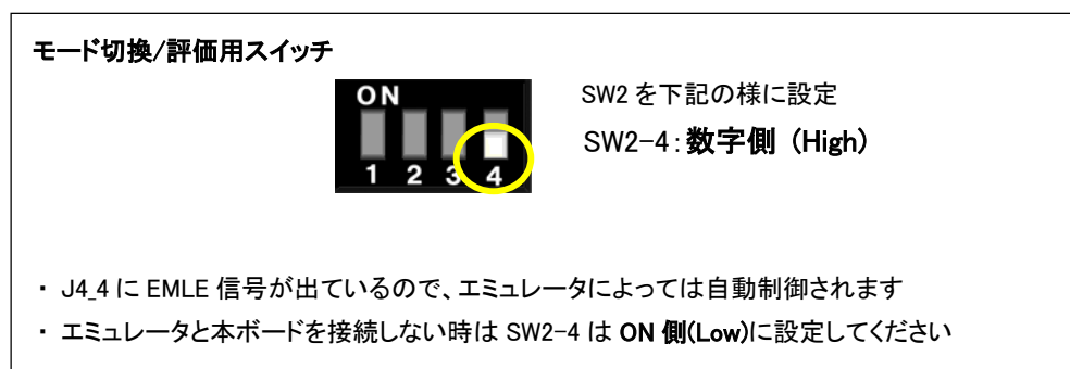
図 2-6 モード切替/評価用スイッチ(SW2)設定図
