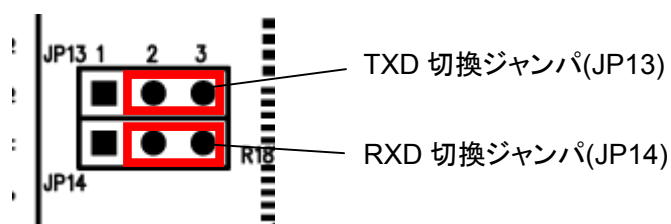
図 2-7 TXD, RXD 切換ジャンパ(JP13, JP14)設定例
