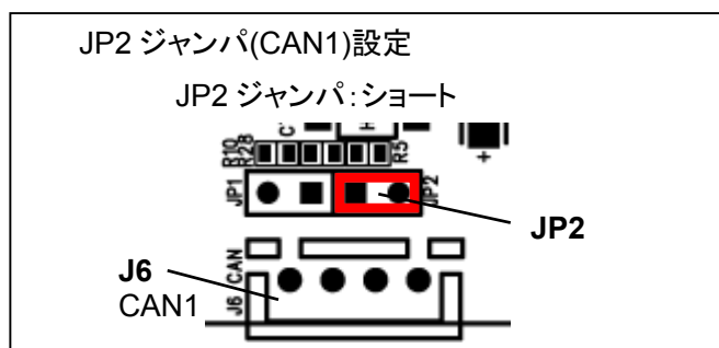
図 2-8 CAN1 終端抵抗イネーブル制御ジャンパ設定図(JP2)
