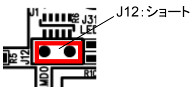
図 2-4 FLMD0 信号切換ジャンパ設定図(J12)
