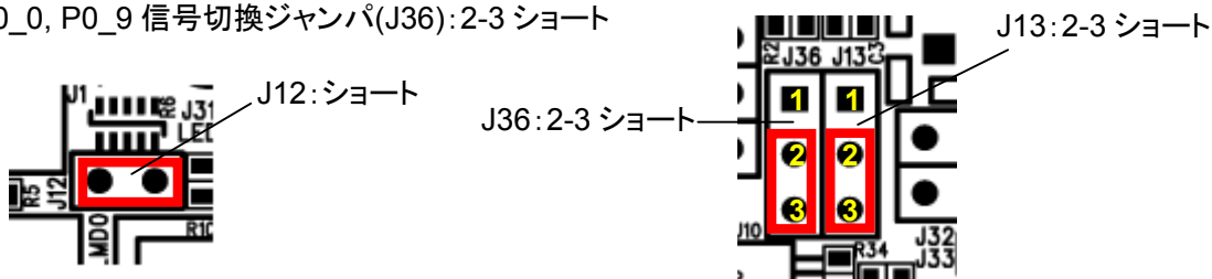
図 2-3 J12, J13, J36 ジャンパ設定図
