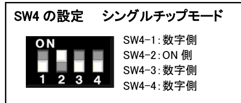
図 3-1 SW4 ジャンパ設定図1
