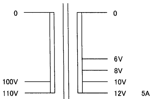
結線図
