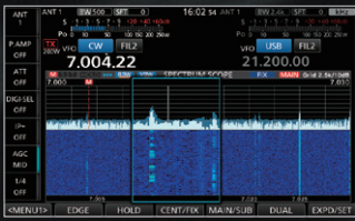
ウォーターフォール（拡大）表示例
