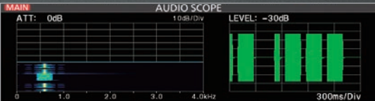
CWキーイング波形表示例
