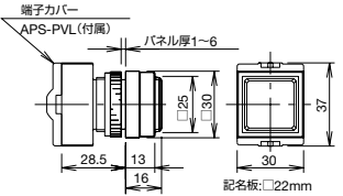
φ22 EB3P-LLW1 / EB3P-LLW2 / EB3P-LLW3形
