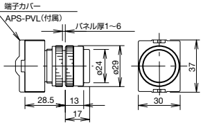
φ22 EB3P-LHW1 / EB3P-LHW2 / EB3P-LHW4形 端子カバー一体型です
