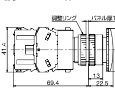
φ22 EB3P-LBAVW411-R形 端子カバー: 一体型
