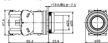
φ22 EB3P-LBAW211 / LBAOW211形 端子カバー: 一体型
