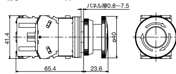
φ22 EB3P-LBH1W110 / LBHA1W110形 端子カバー: 一体型
