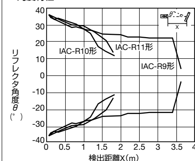
●角度特性
