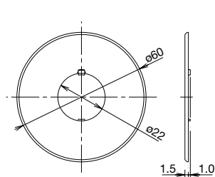
大形 (φ40) ボタン用銘板
