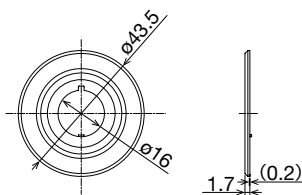
中形(ø30)ボタン用銘板
