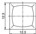
JB-15HLRP2 (AT-4076ボタン装着例)
