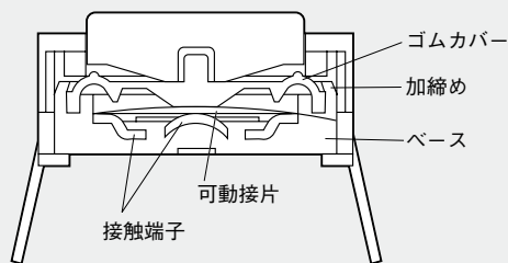
接点部密閉構造
