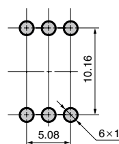
プリント基板取付寸法図 (スイッチ搭載側から見た図)
