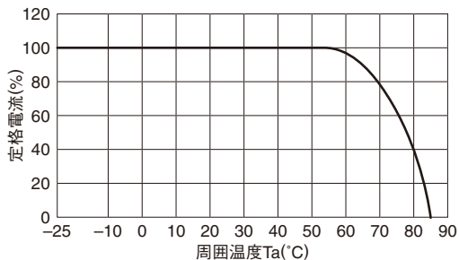
RSHN-2003/2006/2010/2016/2020/2030/ 2040/2050/2060
