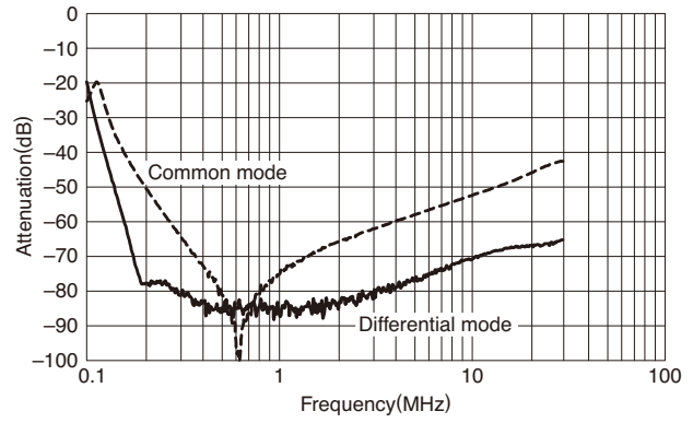
RSHN-2006L
