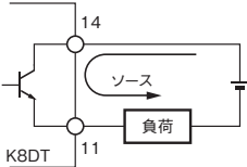
ソース出力用途の場合
