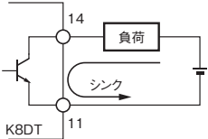
シンク出力用途の場合
