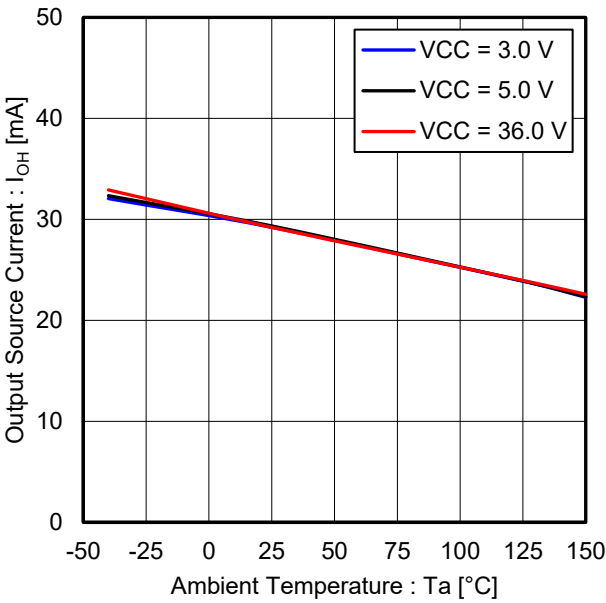
Figure 6. 出力ソース電流 vs 温度 ( V_{OUT} = 0\text{ V} )
