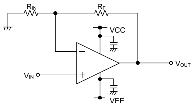
Figure 32. 非反転増幅回路
