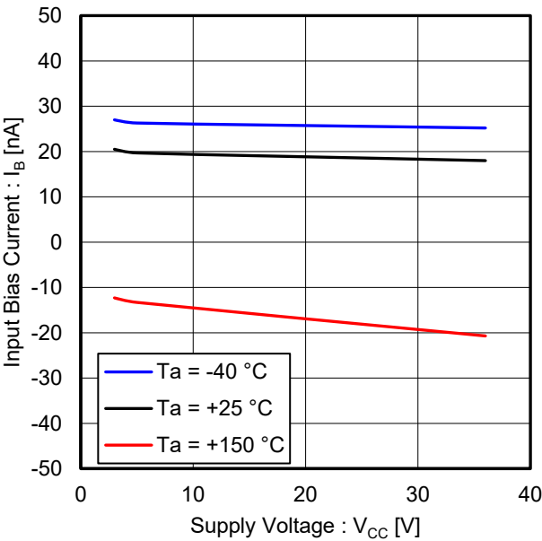
Figure 13. 入力バイアス電流 vs 電源電圧 ( V_{ICM} = V_{CC}/2 )
