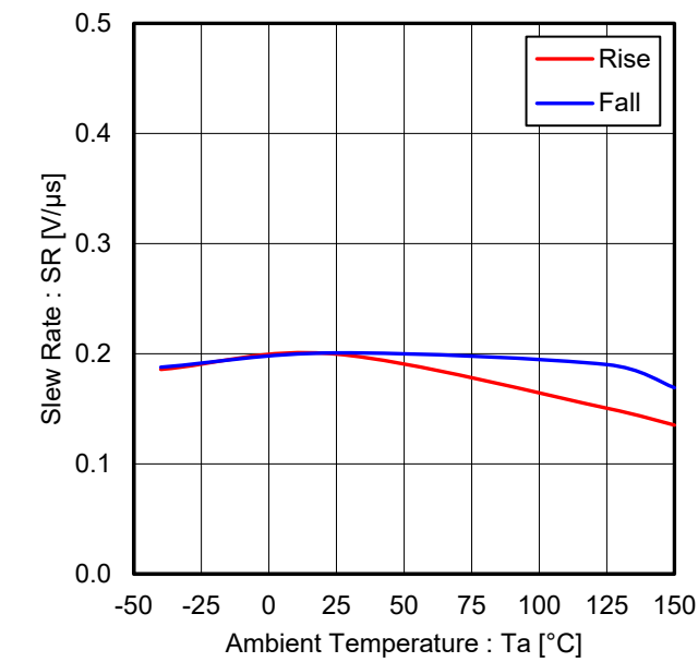
Figure 25. スルーレート vs 温度 ( V_{CC} = 5\text{ V} , R_L = 2\text{ k}\Omega )
