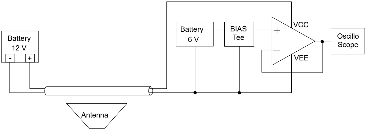
Figure 28. EMI 特性測定回路図
