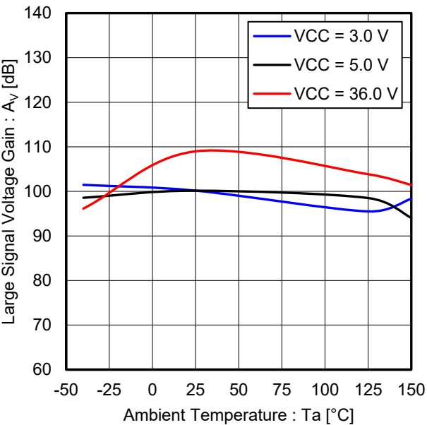
Figure 20. 大振幅電圧利得 vs 温度 ( R_L = 2\text{ k}\Omega )
