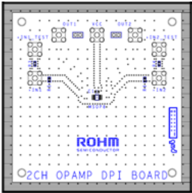
Figure 27. EMI 特性評価ボード
