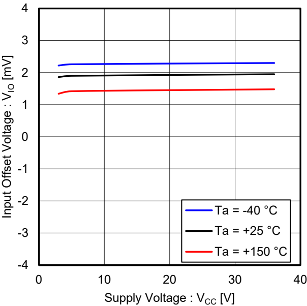
Figure 11. 入力オフセット電圧 vs 電源電圧 ( V_{ICM} = V_{CC}/2 )
