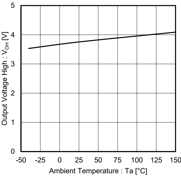
Figure 4. 出力電圧 High vs 温度 ( V_{CC} = 5\text{ V}, R_L = 2\text{ k}\Omega )
