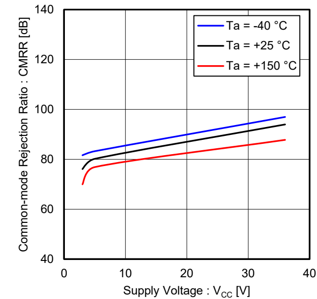
Figure 21. 同相信号除去比 vs 電源電圧 ( V_{OUT} = 1.4\text{ V} )
