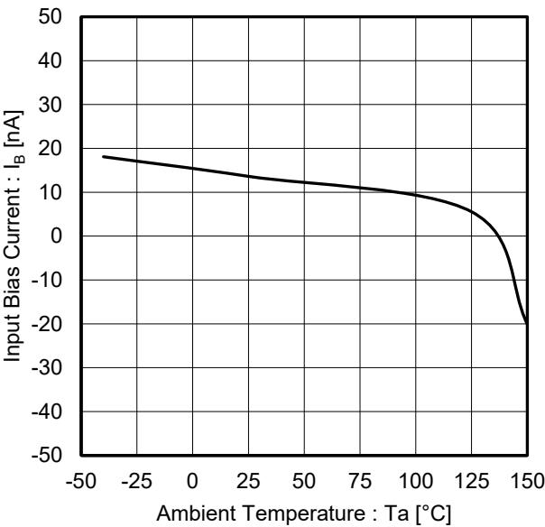
Figure 15. 入力バイアス電流 vs 温度 ( V_{CC} = 30\text{ V} , V_{ICM} = 28\text{ V} , V_{OUT} = 1.4\text{ V} )
