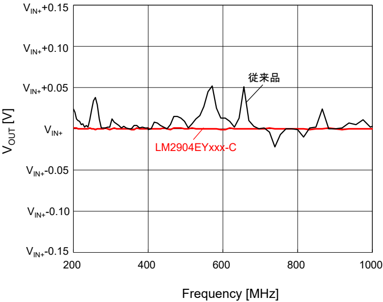
Figure 26. EMI 特性データ
