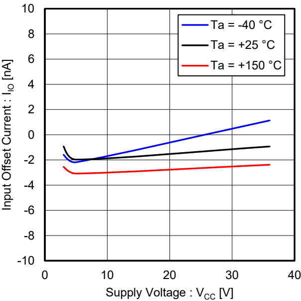
Figure 17. 入力オフセット電流 vs 電源電圧 ( V_{ICM} = V_{CC}/2 )
