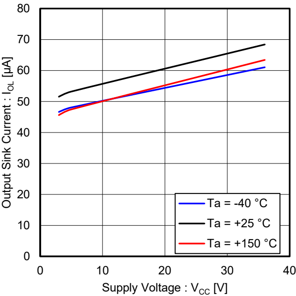
Figure 9. 出力シンク電流 vs 電源電圧 ( V_{OUT} = 0.2\text{ V} )
