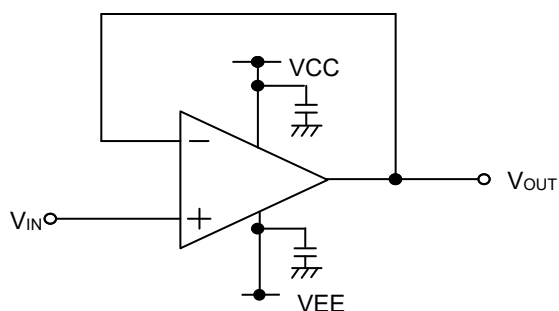
Figure 30. ボルテージフォロワ回路
