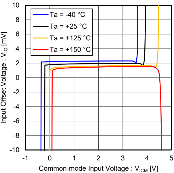
Figure 16. 入力オフセット電圧 vs 同相入力電圧範囲 ( V_{CC} = 5\text{ V} )
