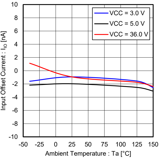
Figure 18. 入力オフセット電流 vs 温度 ( V_{ICM} = V_{CC}/2 )
