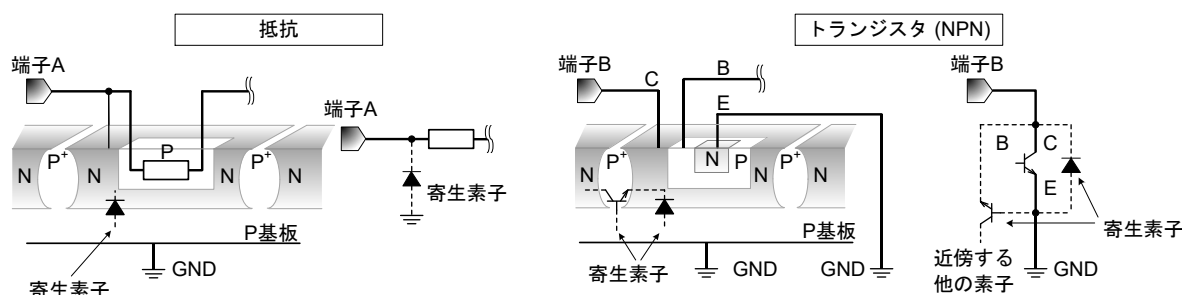
Figure 33. モノリシック IC 構造例
