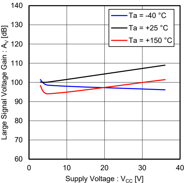
Figure 19. 大振幅電圧利得 vs 電源電圧 ( R_L = 2\text{ k}\Omega )
