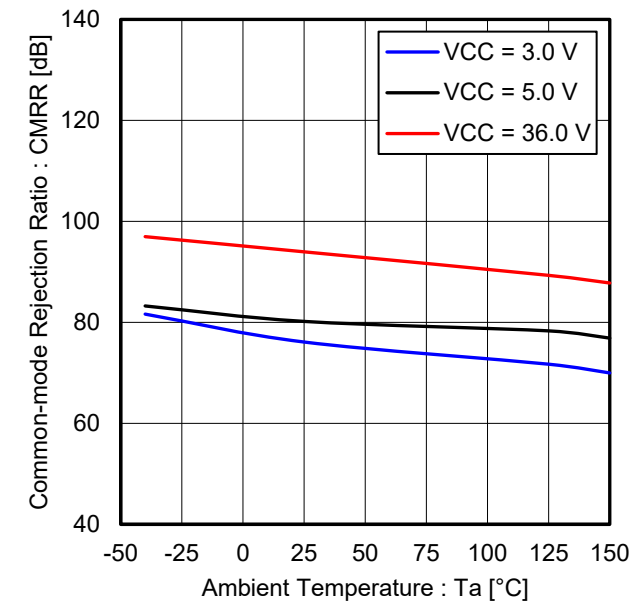
Figure 22. 同相信号除去比 vs 温度 ( V_{OUT} = 1.4\text{ V} )
