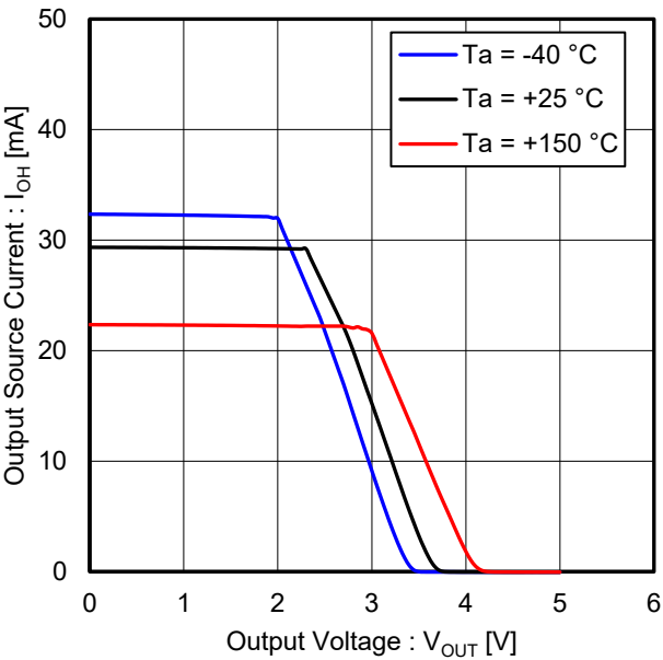
Figure 5. 出力ソース電流 vs 出力電圧 ( V_{CC} = 5\text{ V} )
