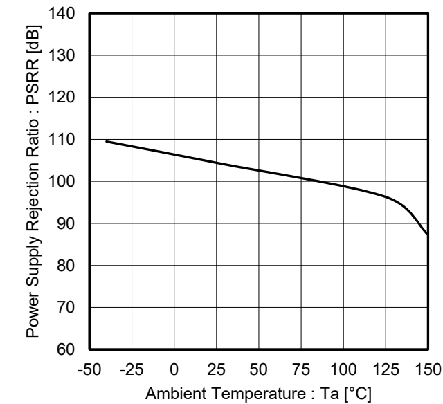
Figure 23. 電源電圧除去比 vs 温度 ( V_{CC} = 5\text{ V} )
