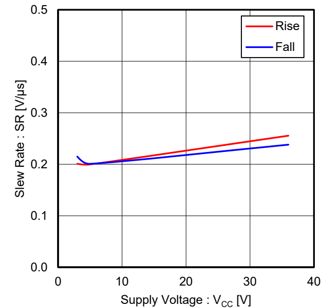
Figure 24. スルーレート vs 電源電圧 ( T_a = 25\text{ }^{\circ}\text{C} , R_L = 2\text{ k}\Omega )
