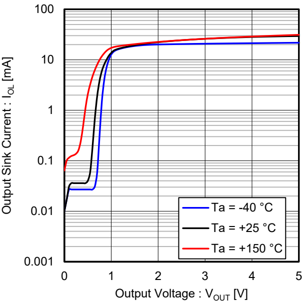
Figure 7. 出力シンク電流 vs 出力電圧 ( V_{CC} = 5\text{ V} )
