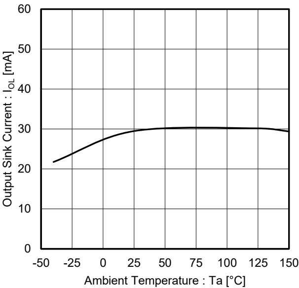
Figure 8. 出力シンク電流 vs 温度 ( V_{CC} = 5\text{ V} , V_{OUT} = 5\text{ V} )
