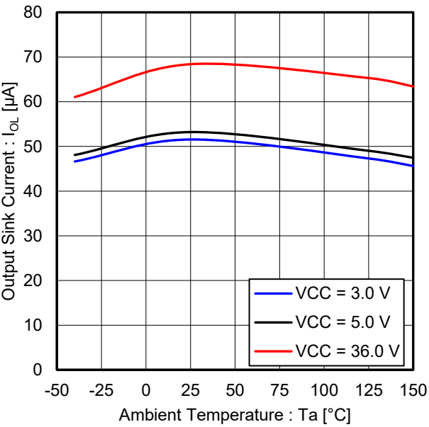
Figure 10. 出力シンク電流 vs 温度 ( V_{OUT} = 0.2\text{ V} )
