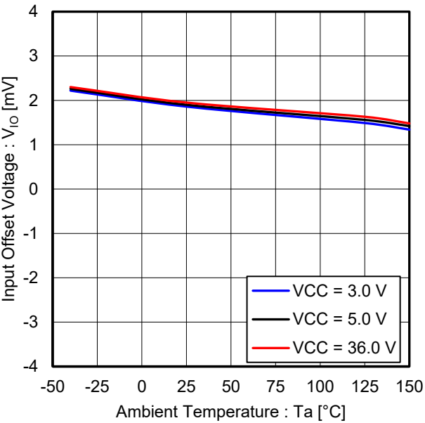
Figure 12. 入力オフセット電圧 vs 温度 ( V_{ICM} = V_{CC}/2 )
