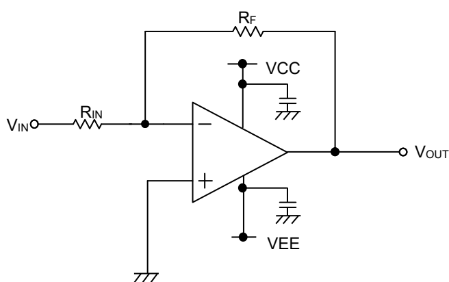
Figure 31. 反転増幅回路
