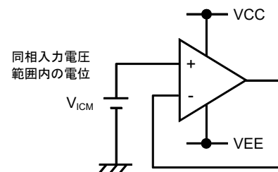
Figure 29. 未使用回路の処理例
