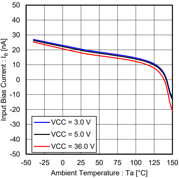
Figure 14. 入力バイアス電流 vs 温度 ( V_{ICM} = V_{CC}/2 )
