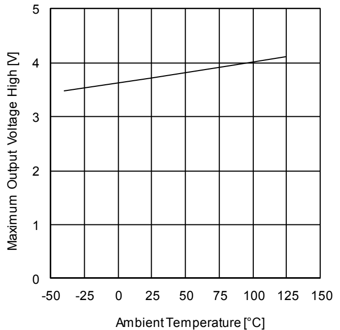
Figure 4. 最大出力電圧(High)－温度特性 (V cc =5V, R L =10kΩ)
