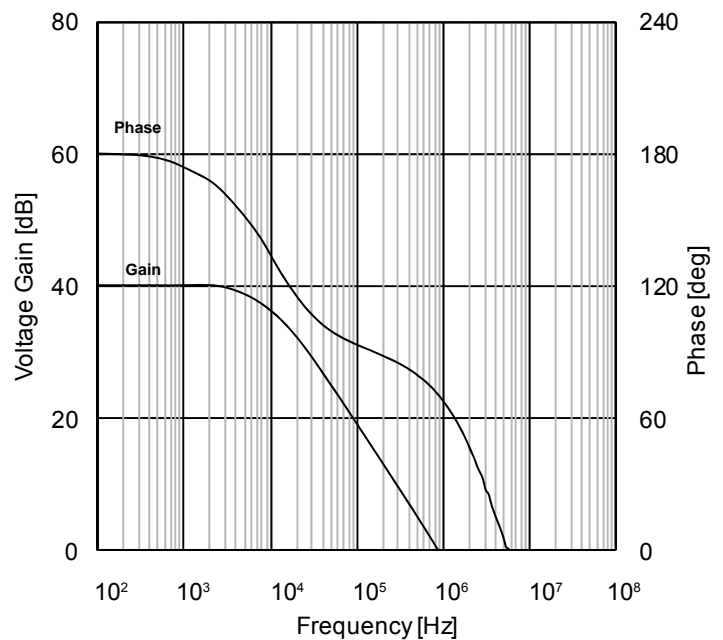
Figure 24. 電圧利得・位相一周波数特性 (V CC =30V, R L =2kΩ, C L =100pF)
