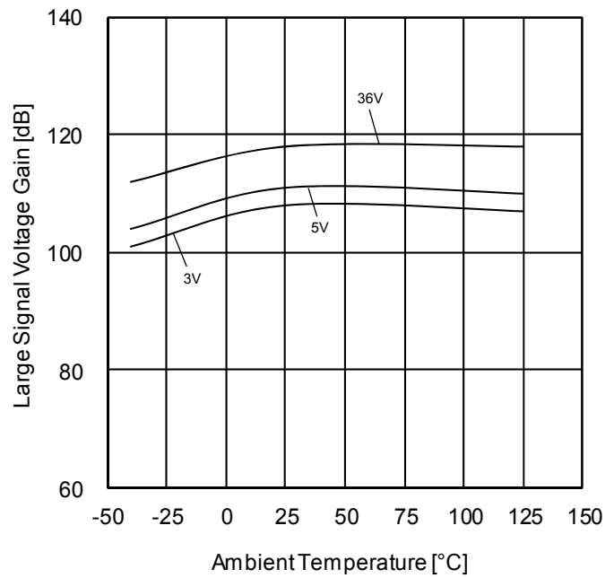
Figure 55. 大振幅電圧利得—温度特性 (R L =2kΩ)
