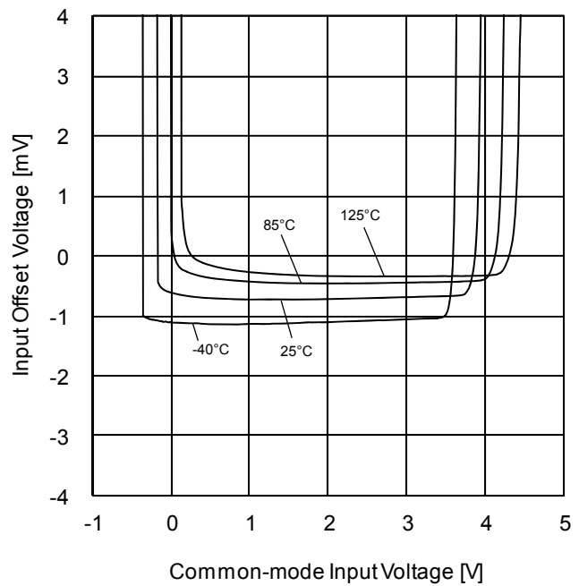
Figure 47. 入力オフセット電圧—同相入力電圧特性 ( V_{CC}=5V )
