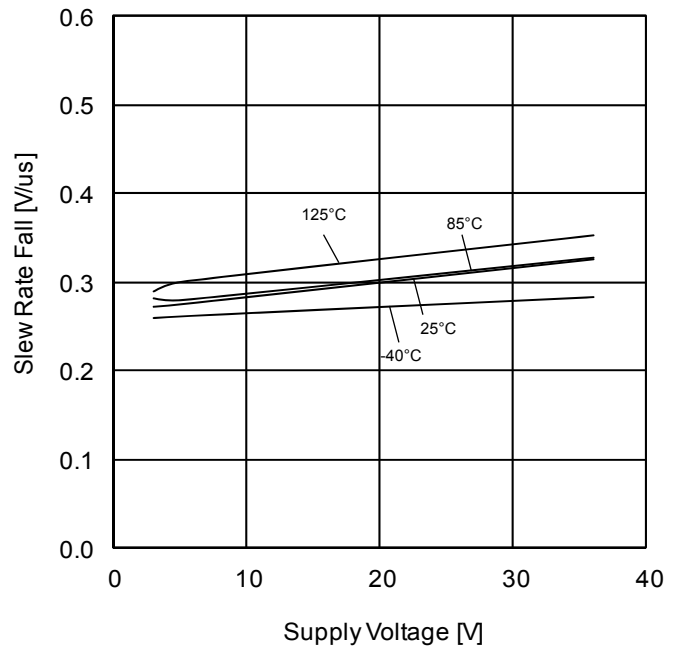
Figure 22. スルーレート(H-L)–電源電圧特性 (R L =2kΩ)
