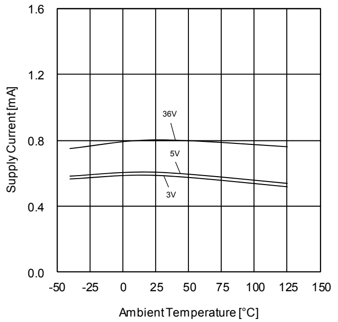
Figure 2. 回路電流－温度特性
