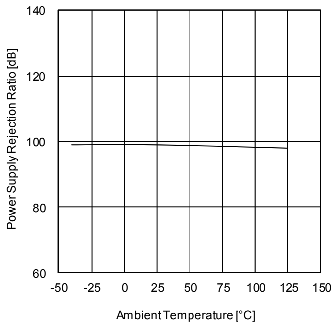
Figure 58. 電源電圧除去比—温度特性
