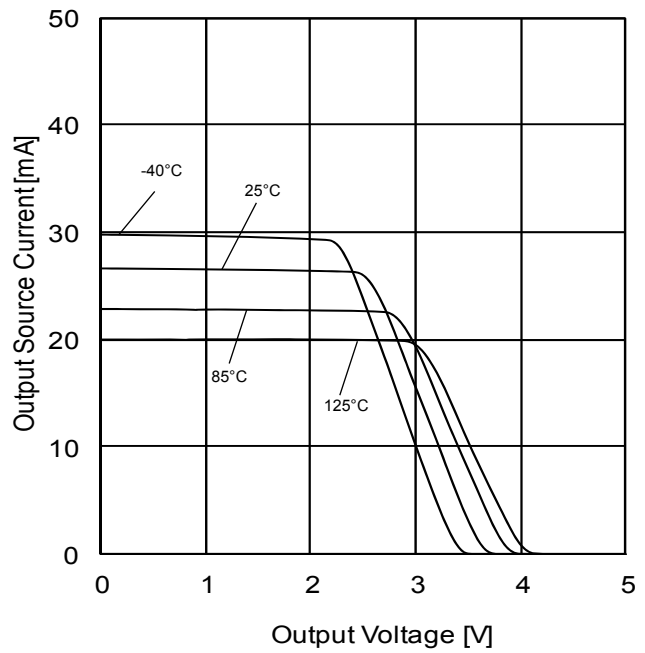
Figure 6. 出カソース電流－出力電圧特性 ( V_{CC}=5V )
