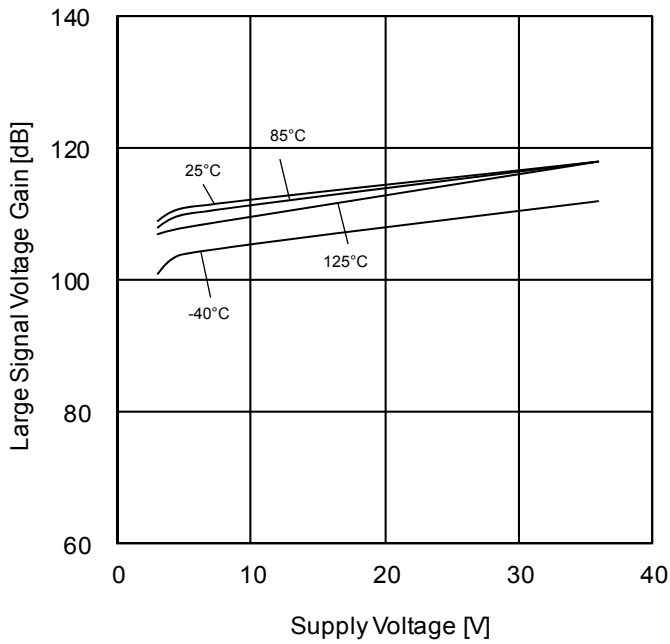
Figure 54. 大振幅電圧利得—電源電圧特性 (R L =2kΩ)
