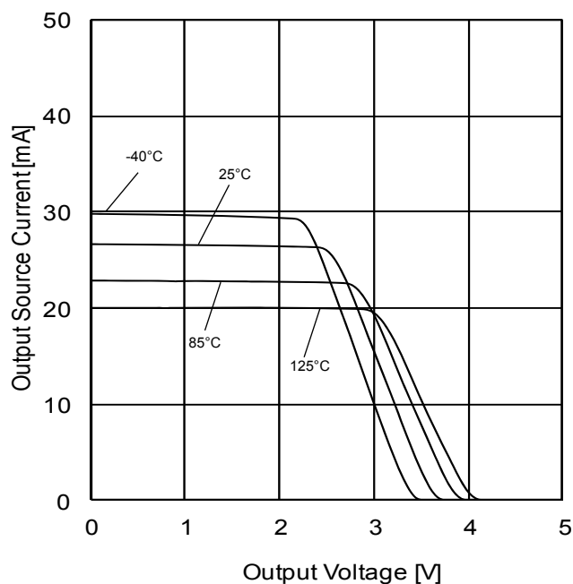
Figure 35. 出力ソース電流－出力電圧特性 ( V_{CC}=5V )
