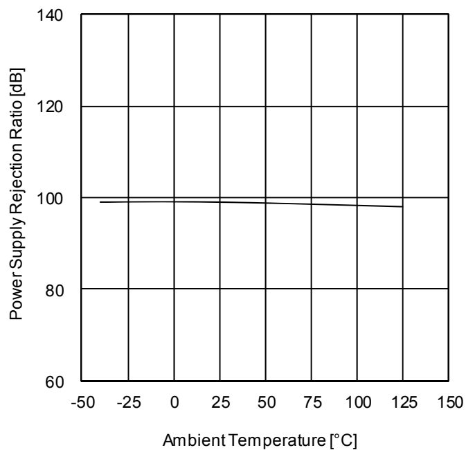
Figure 29. 電源電圧除去比—温度特性
