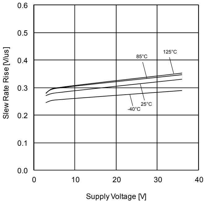
Figure 21. スルーレート(L-H)–電源電圧特性 (R L =2kΩ)
