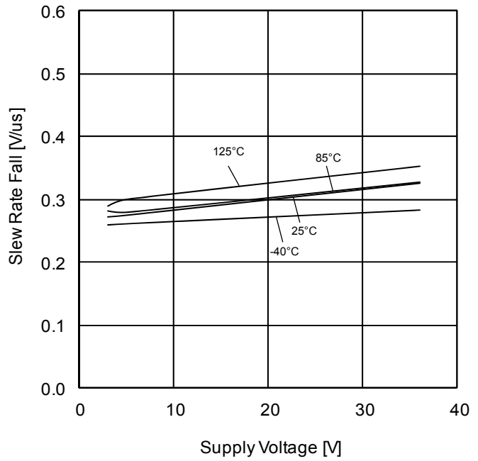
Figure 51. スルーレート(H-L)–電源電圧特性 (R L =2kΩ)
