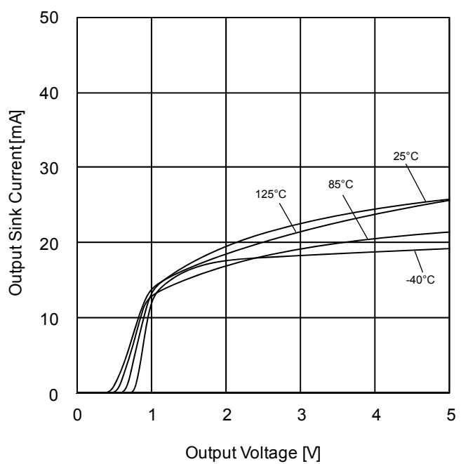
Figure 8. 出カシンク電流－出力電圧特性 ( V_{CC}=5V )
