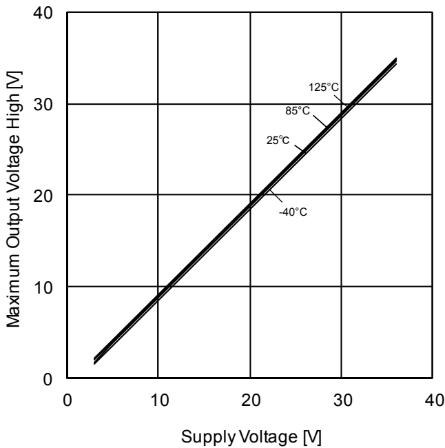
Figure 3. 最大出力電圧(High)－電源電圧特性 (R L =10kΩ)
