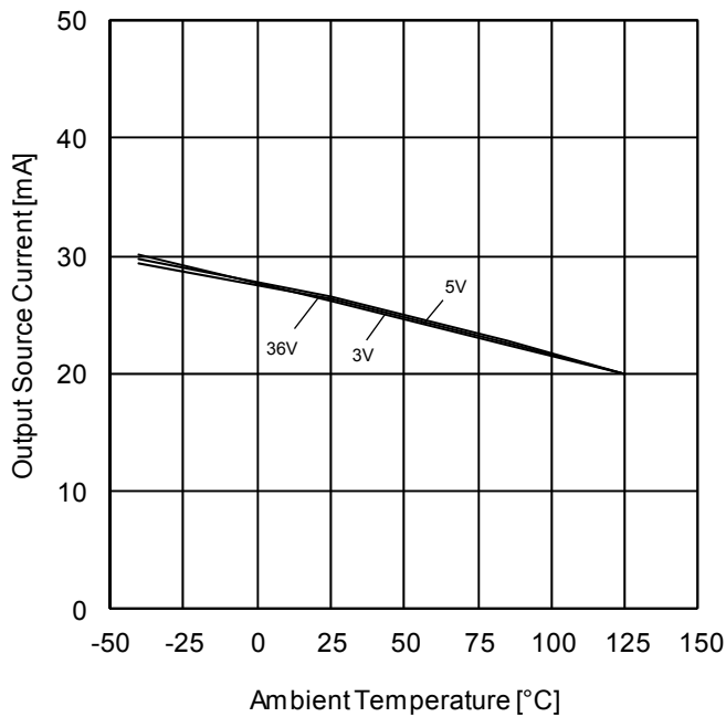
Figure 7. 出カソース電流－温度特性 ( V_{OUT}=0V )
