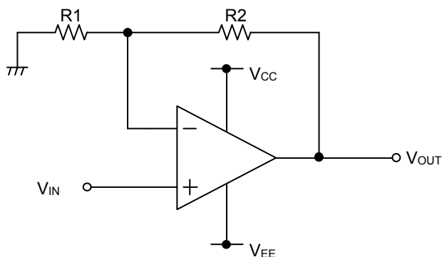
Figure 66. 非反転増幅回路
