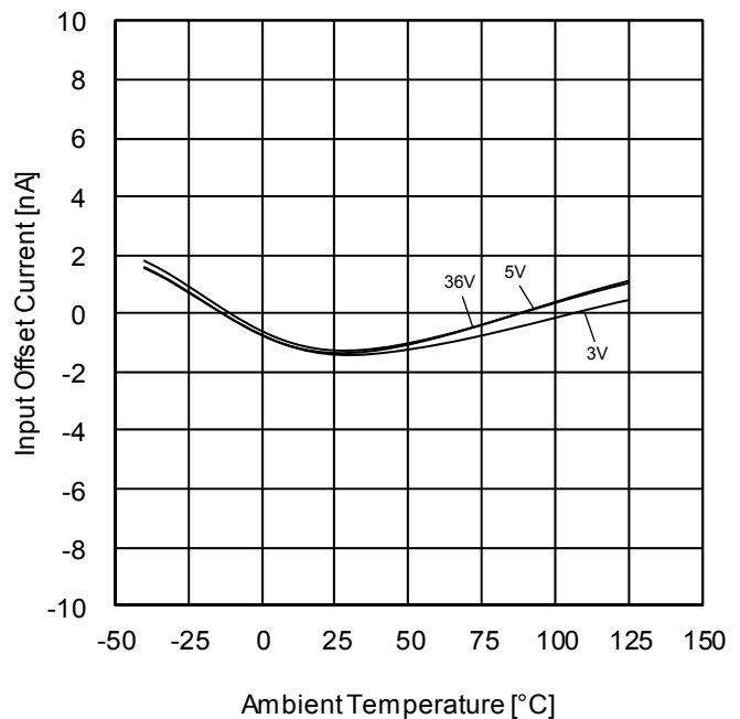
Figure 49. 入力オフセット電流—温度特性 ( V_{ICM}=V_{CC}/2 , E_K=-V_{CC}/2 )
