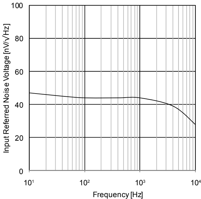
Figure 52. 入力換算雑音電圧–周波数特性 (V CC =5V)
