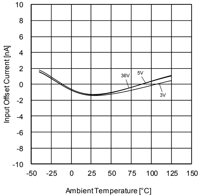
Figure 20. 入力オフセット電流—温度特性 ( V_{ICM}=V_{CC}/2 , E_K=-V_{CC}/2 )
