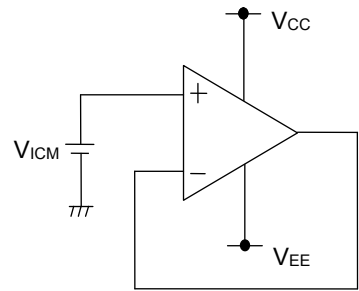
Figure 63. 未使用回路処理例
