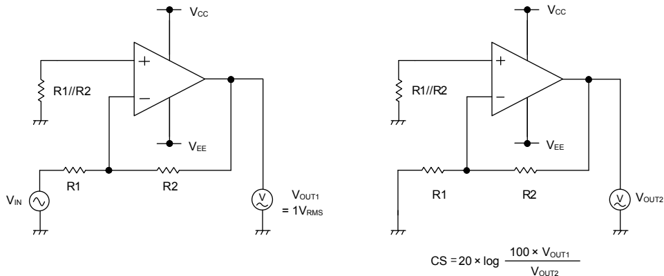
Figure 62. 測定回路 3 (チャンネルセパレーション) (R1=1kΩ,R2=100kΩ)
