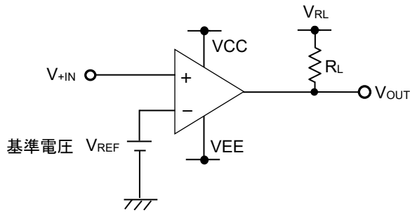
Figure 21. -IN を基準とした場合の回路例
