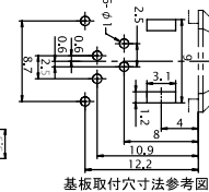
基板取付穴寸法参考図 t1.0 または t1.6
