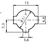
パネル取付穴寸法参考図 Mounting Hole (t1.6)
