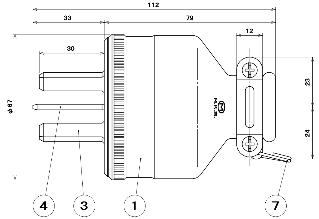
ゴムボデーを外した状態
