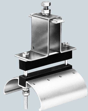
E-600型(ブラケット70R)
