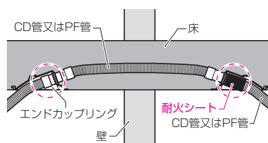
■サブウェイ工法(KK27-015号)
