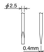
図2. 適用取りはずし工具寸法
