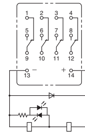
形MY4(Z) IN-D2(S) (DC仕様のみ)
