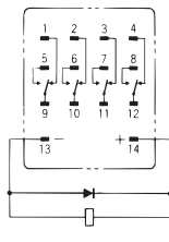
形MY4Z-D (DC仕様のみ)
