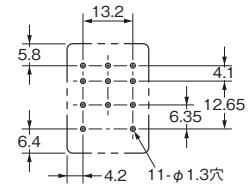
プリント基板加工寸法
