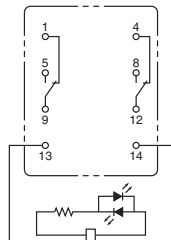
形MY2IN(S) (AC仕様)
