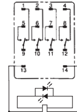
形MY4ZN-CR (AC仕様のみ)
