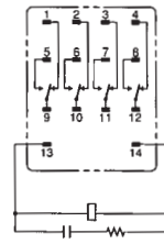
形MY4Z-CR (AC仕様のみ)
