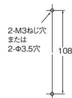
取り付け穴加工寸法
