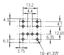
プリント基板加工寸法 (BOTTOM VIEW)
