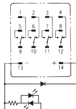
形MY4ZN-D2 (DC仕様のみ)
