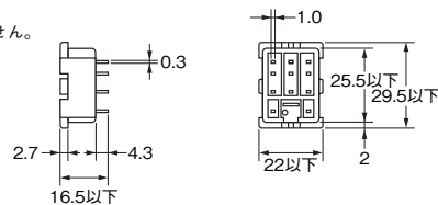
端子配置/内部接続図
