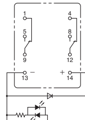
形MY2IN-D2(S) (DC仕様のみ)
