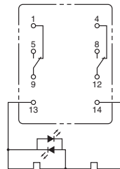
形MY2IN(S) (DC仕様)
