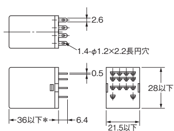
形MY4Z-D (DC仕様のみ)
