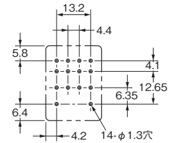
プリント基板加工寸法
