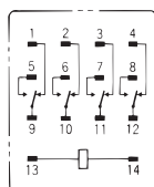
端子配置/内部接続図 (BOTTOM VIEW) 形MY4Z (AC/DC仕様)
