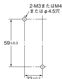
取り付け穴加工寸法
