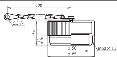
プラグキャップ：NCS-54-PCa
