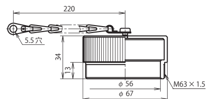
プラグキャップ：NCS-60-PCa
