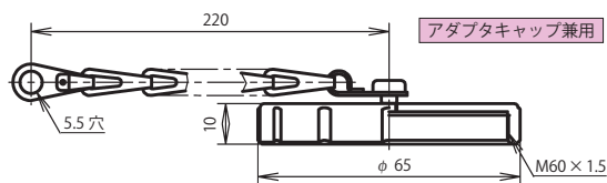
レセプタクルキャップ：NCS-54-RCa
