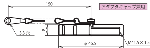
レセプタクルキャップ：NCS-40-RCa
