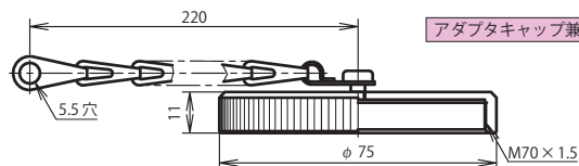
レセプタクルキャップ：NCS-64-RCa
