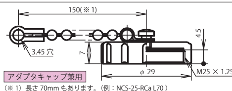
レセプタクルキャップ: NCS-25-RCa
