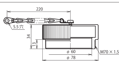
プラグキャップ：NCS-64-PCa
