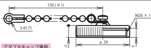
プラグキャップ：NJC-24-PCa
