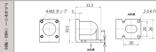
NJC-16 ヨウ L ザ
