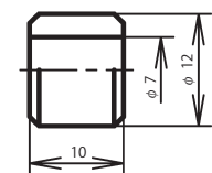
ケーブルブッシング：CBAS-12-7
