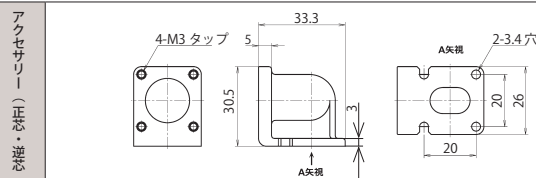
NJC-16 用ヨウ L ザ
