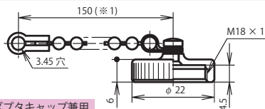
レセプトクルキャップ：NJC-16-RCa
