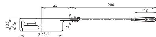
プラグ防水キャップ：NRW-28-PCa・1
