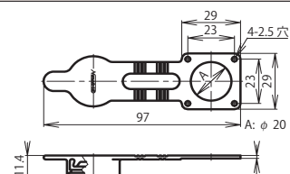
レセプタクル防水キャップ: NRW-20-RCa・1
