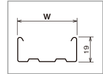
適合Mバー寸法
