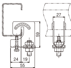
専用座金
