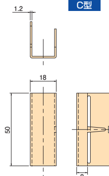
下穴10×20
