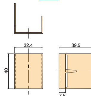
下穴10×35
