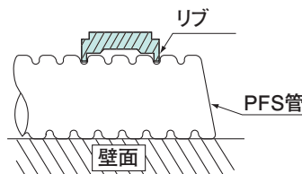
取付断面図 (PFS管)
