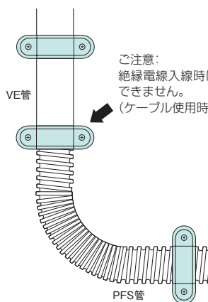
取付断面図 (PFS管)
