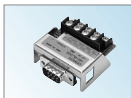
RS-232C/RS-422A変換ユニット 形NS-AL002
