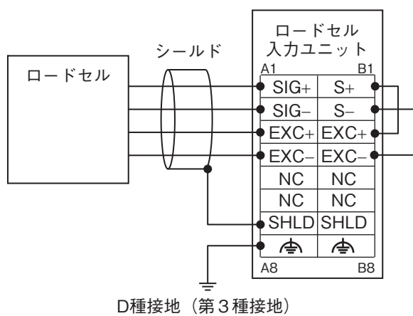
4線式ロードセルとの接続図
