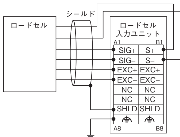
6線式ロードセルとの接続図
