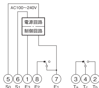
形61F-LS-CP08-A
