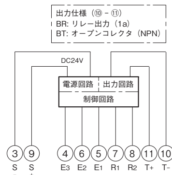
形61F-LS-CP11-B
