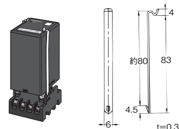
形PFC-N8
