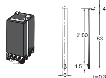
形PFC-N8
