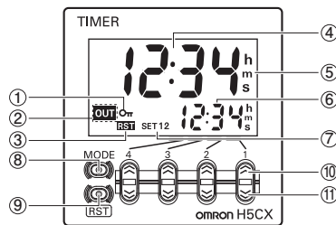
(正面図)
